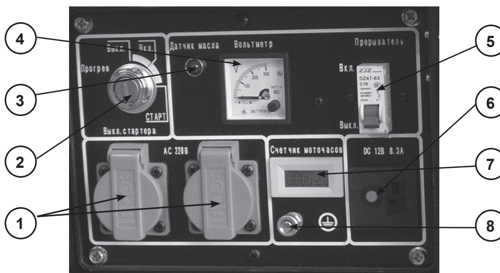
1. Розетки 220В 2. Замок зажигания 3. Контрольная лампочка датчика масла 4. Вольметр 5. Прерыватель напряжения генератора 6. Розетка 12В с аварийным выключателем 7. Счетчик моточасов 8. Клемма подключения заземления.
