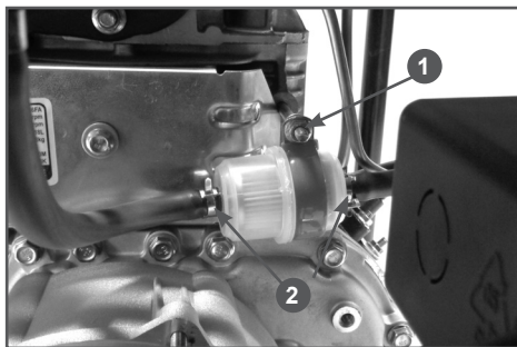
Рис. 14 Замена топливного фильтра
