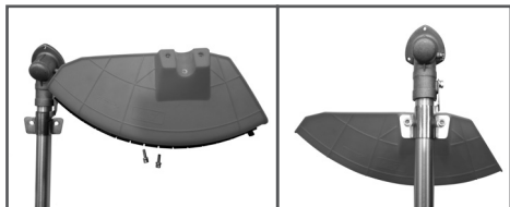
Рис.2 Установка защитного кожуха
